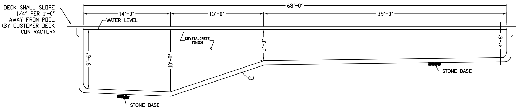
SECTION B-B SCALE: 1/8" = 1'-0"
