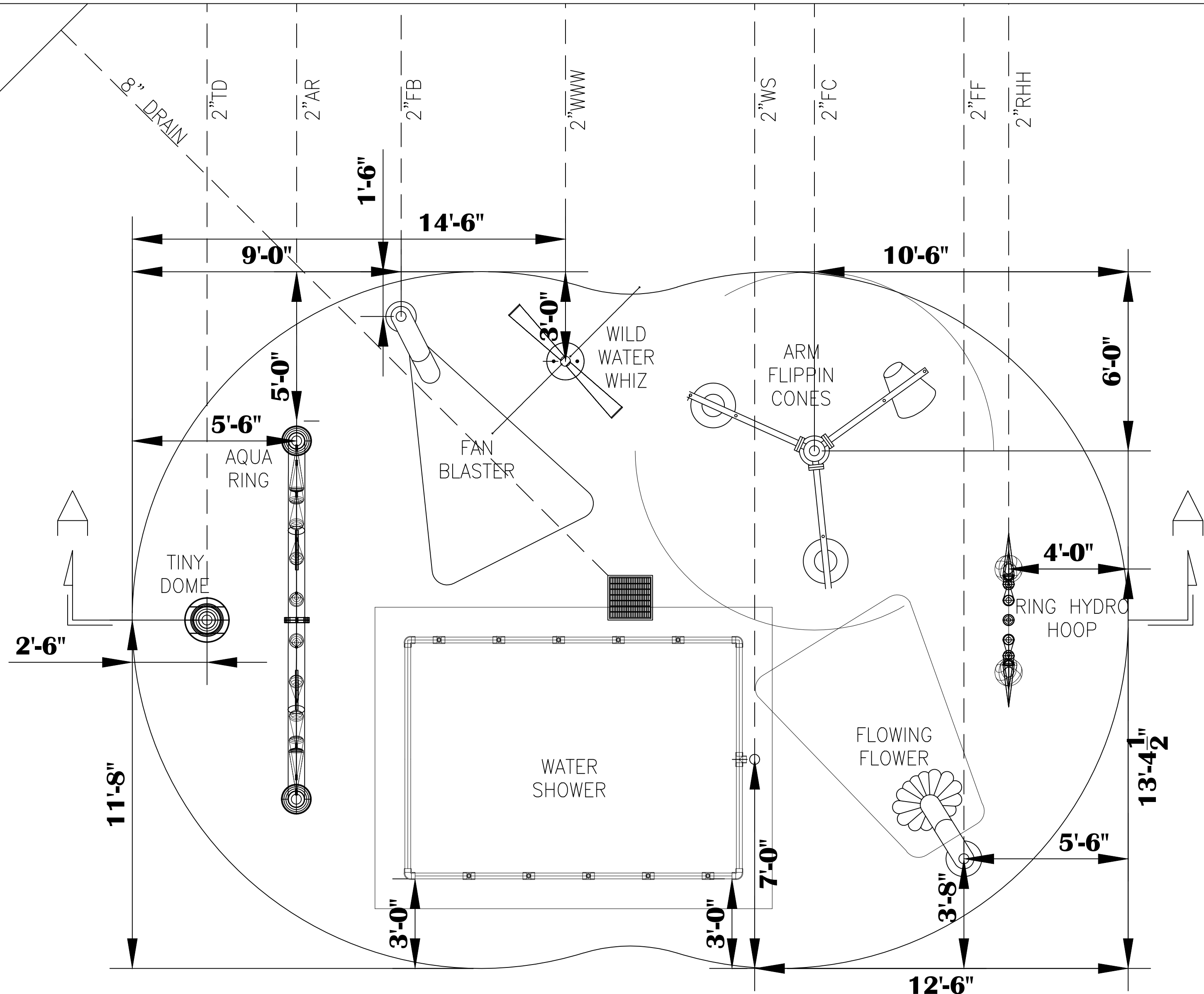
PAD PLAN SCALE: 3/8" = 1'-0"
