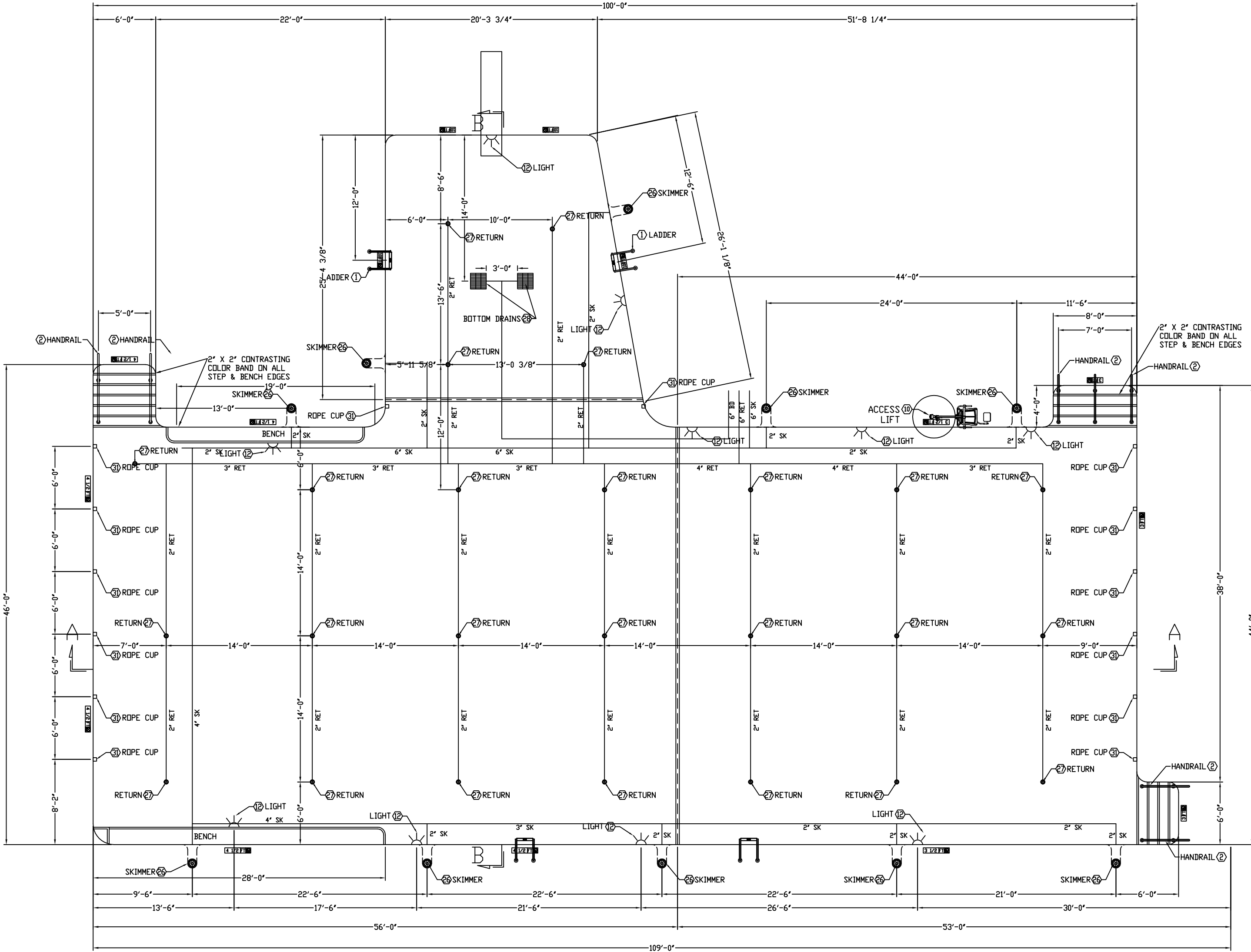
POOL PLAN SCALE: 1/8" = 1'-0"
